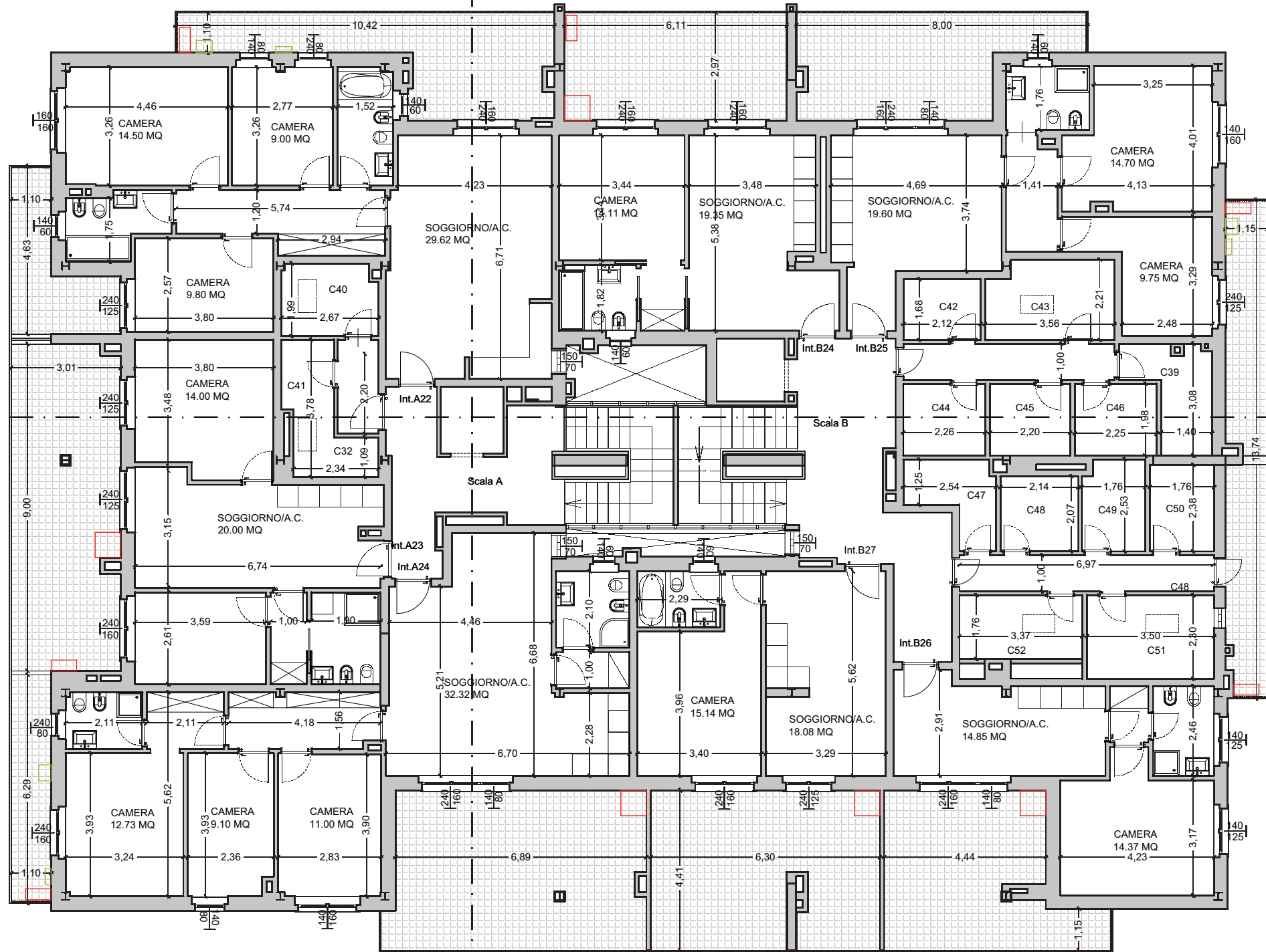
PIANTA PIANO SESTO SC. 1:100
