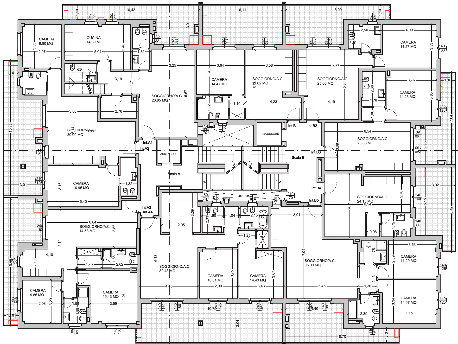
PIANTA PIANO PRIMO SC. 1:100
