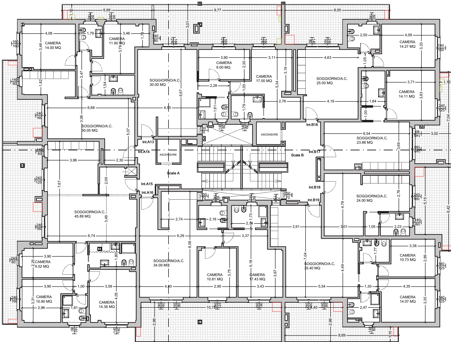
PIANTA PIANO QUARTO SC. 1:100
